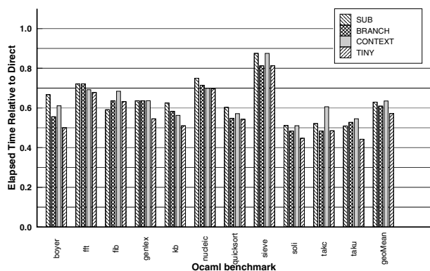
(b) OCaml PPC970 elapsed (real) sec
